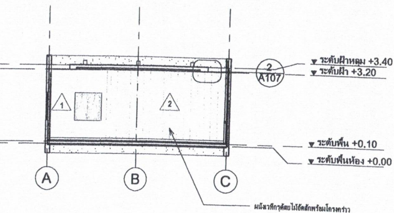
2 Section 2 1 : 100
