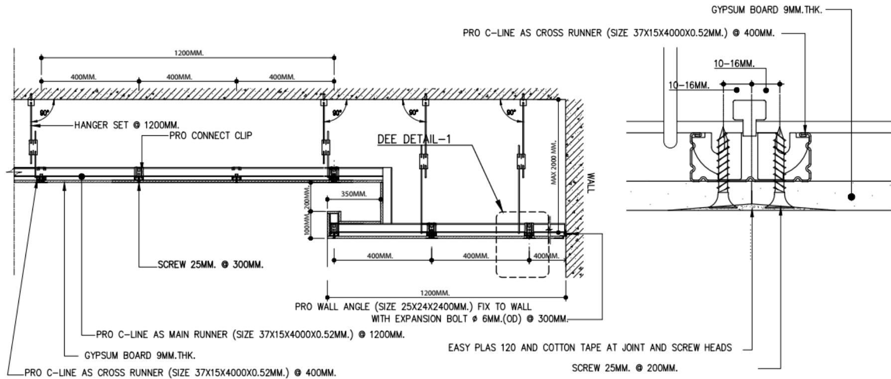
DETAIL-1 SCALE 1 : 1
