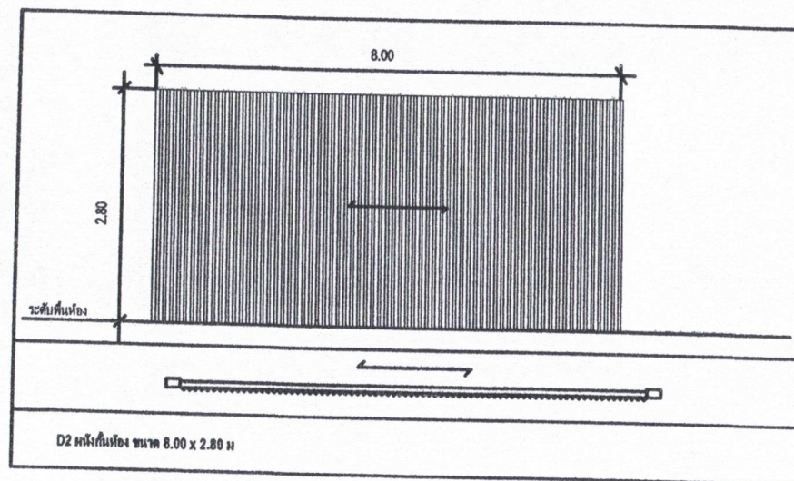
แบบขยายประตู D2 1 : 50
